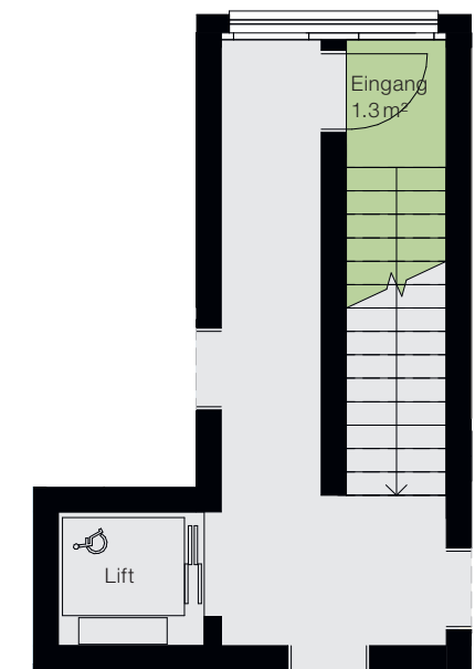
2. Obergeschoss
